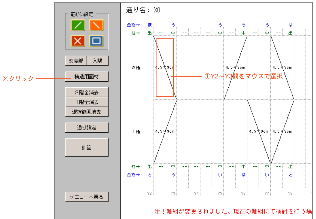
図3.3.5 面材の設定
