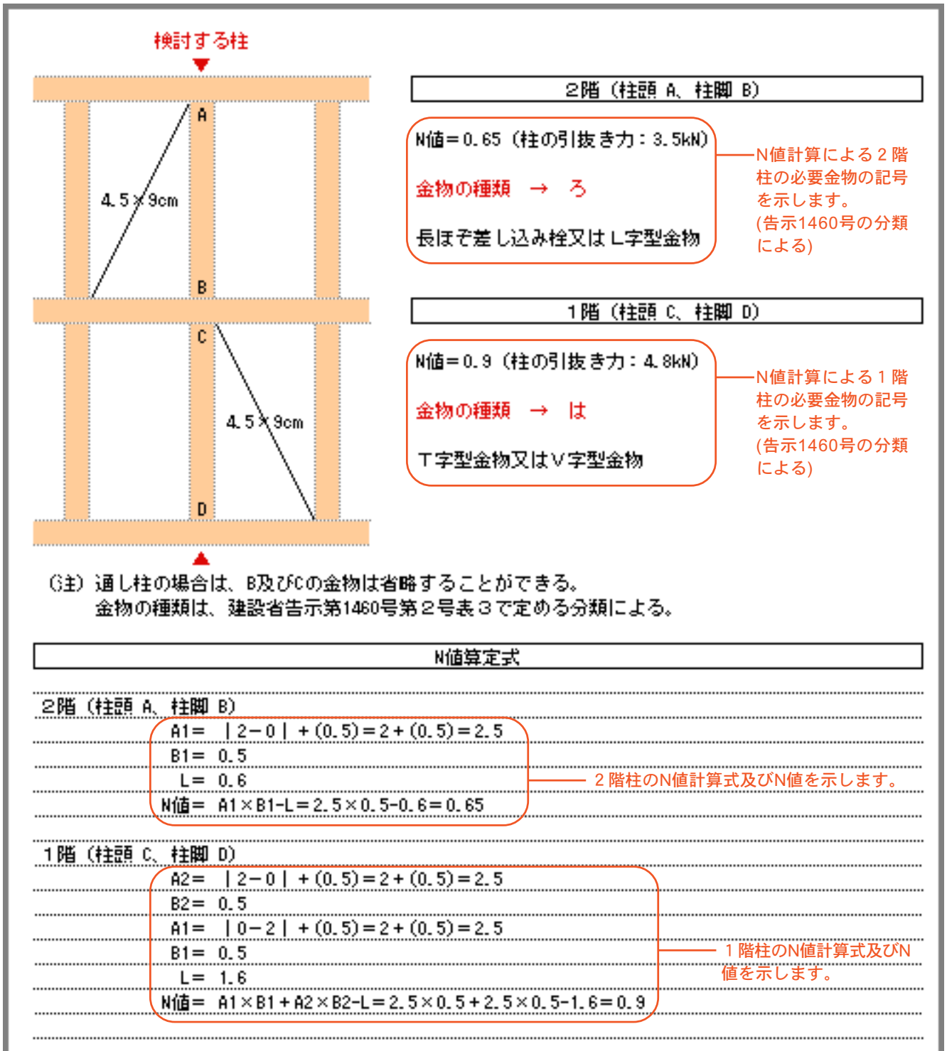
図4.1.6 「モデルプランのX0通りY6」の計算結果
